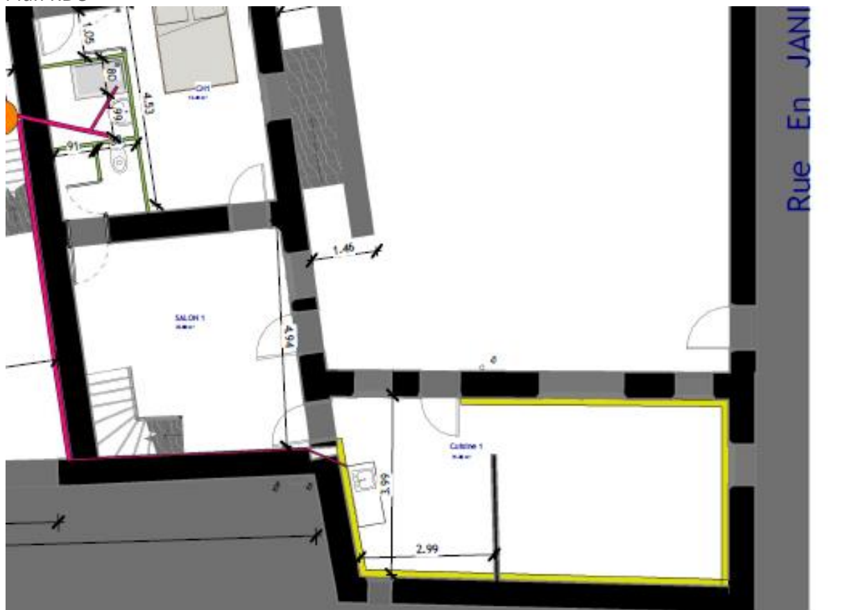
Plan étage
